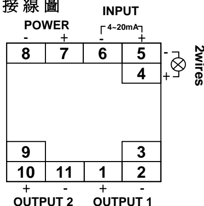
接線圖
