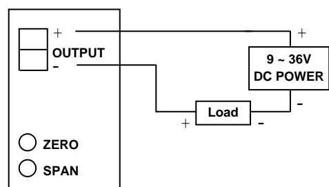
接線圖
